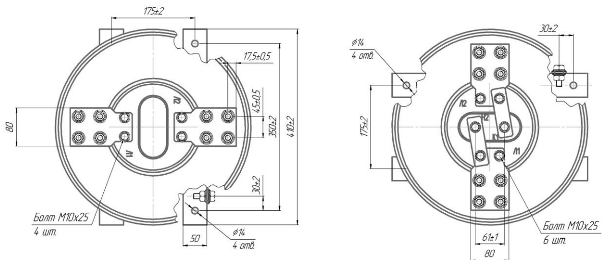
Рис. 2 (Исполнение трансформатора с двумя первичными токами) Остальное см. рис. 1 A
