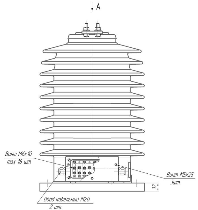
Рис. 2 (Исполнение трансформатора с двумя первичными токами) Остальное см. рис. 1
