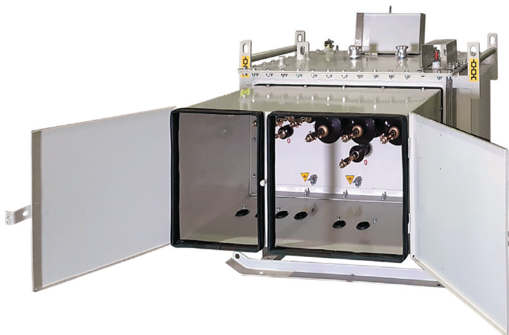
Трансформатор герметичный, без расширителя ТМПНГ-СЭЩ
